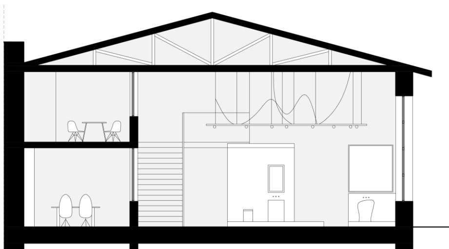
PRZEKRÓJ POPRZECZNY
